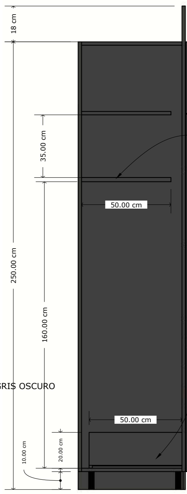
VISTA LATERAL IZQUIERDA MUEBLE 01
