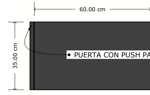
VISTA LATERAL
