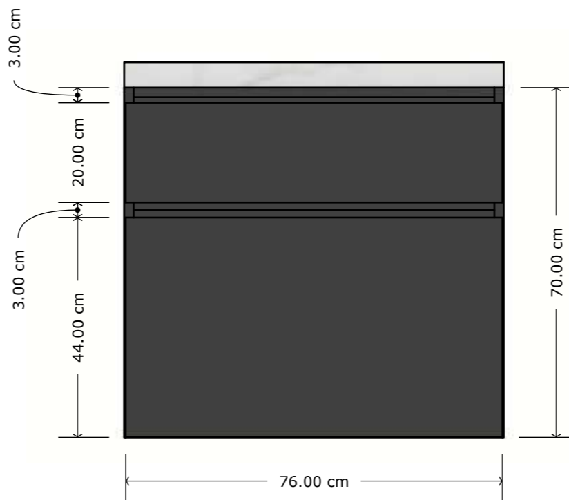
VISTA FRONTAL (3)
