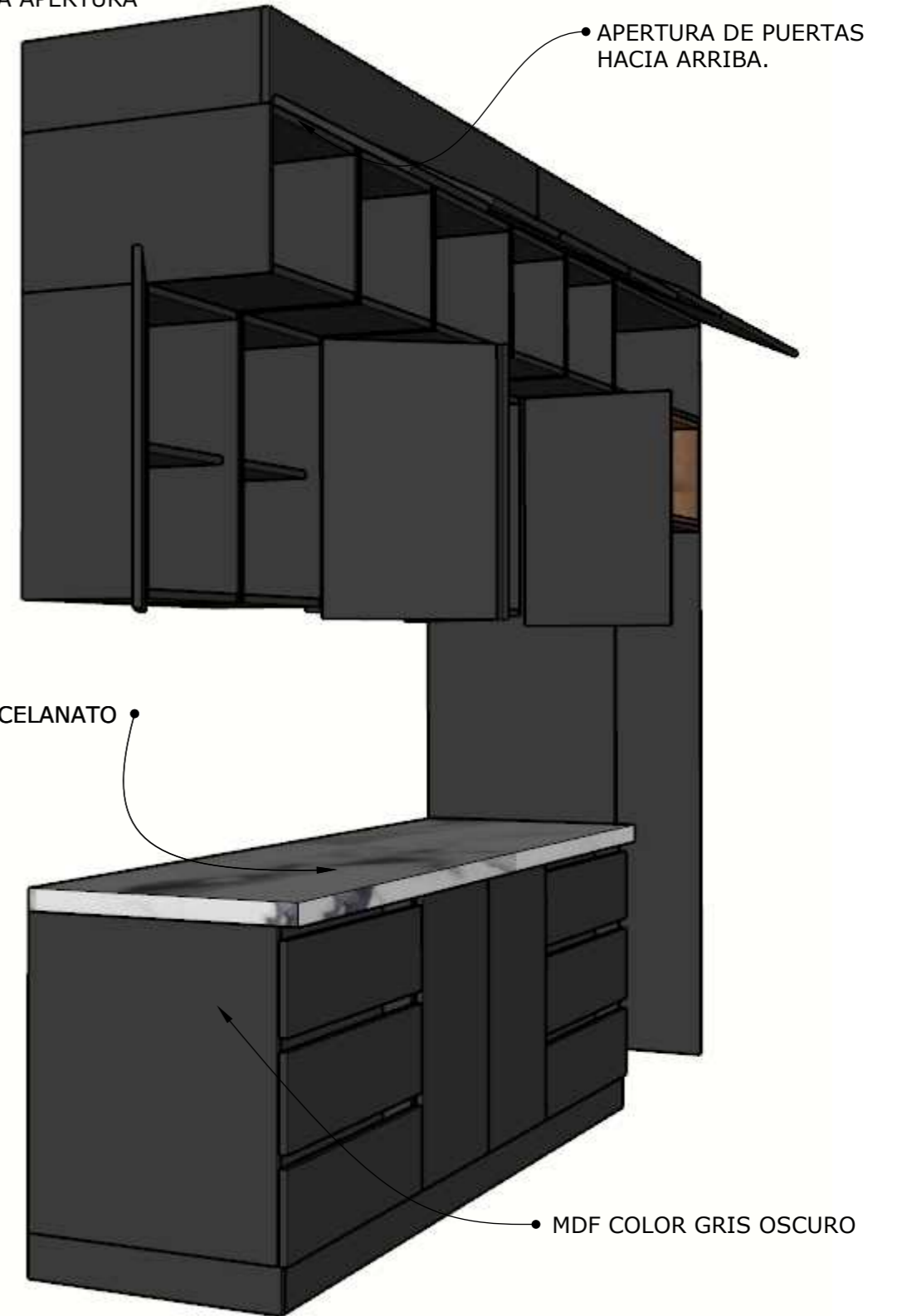
VISTA APERTURA DE PUERTAS
