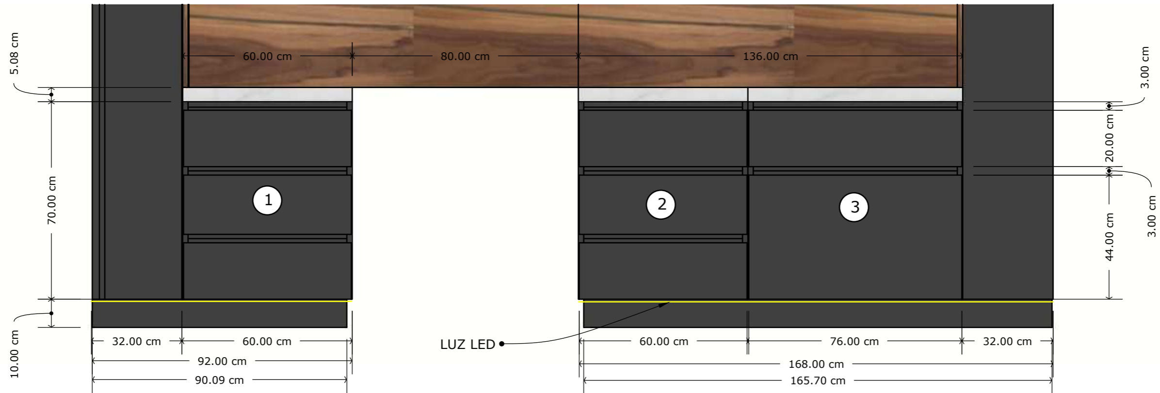
VISTA FRONTAL - FUNCIONAMIENTO Y DIMENSIONES DE GAVETAS
