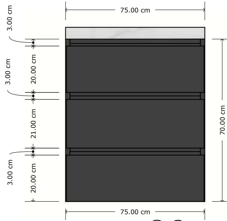
VISTA FRONTAL (4) (6)
