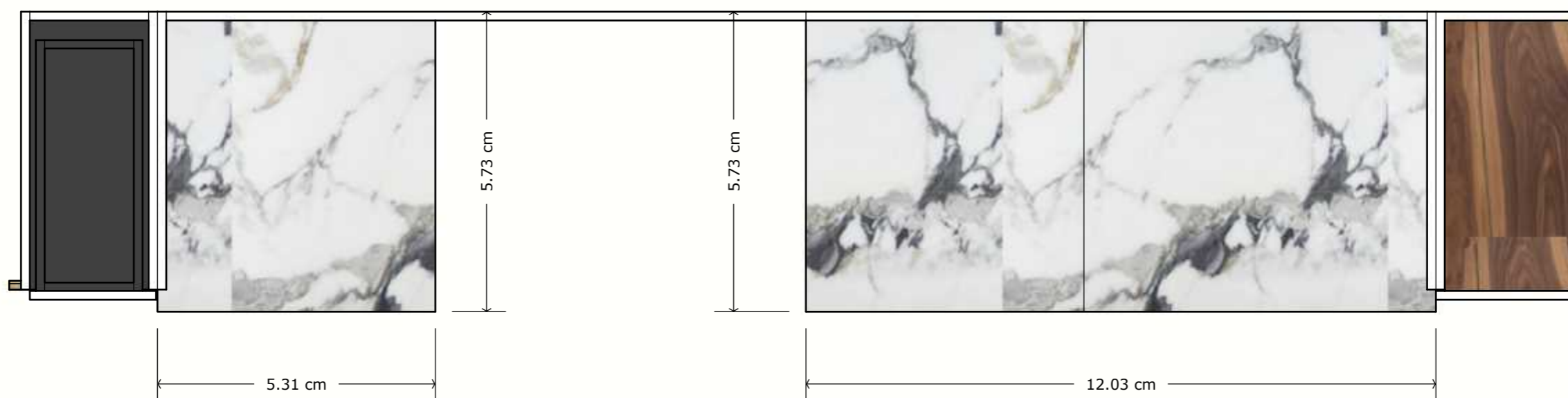
VISTA EN PLANTA MUEBLE 01 TOP DE PORCELANATO
