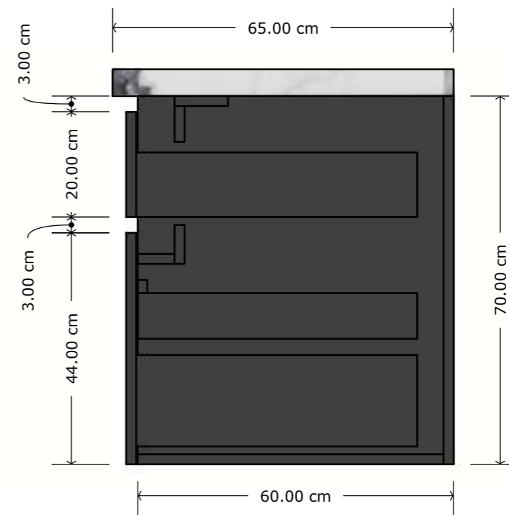
VISTA LATERAL (3)
