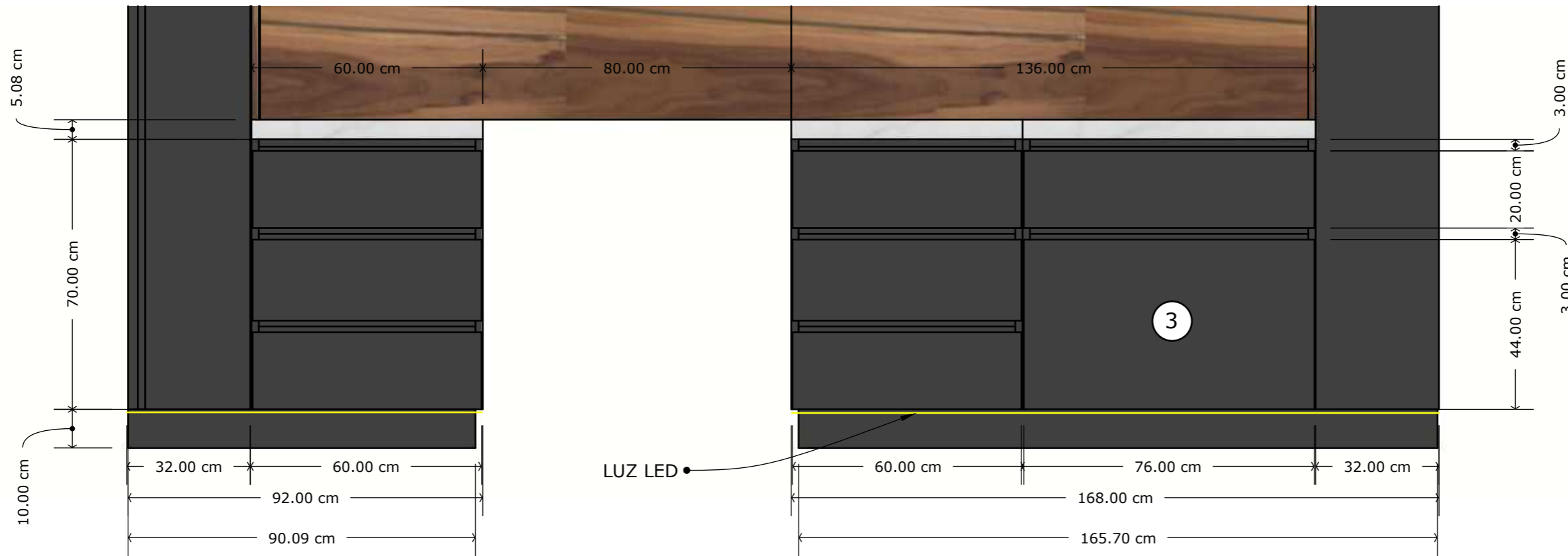
VISTA FRONTAL - FUNCIONAMIENTO Y DIMENSIONES DE GAVETAS
