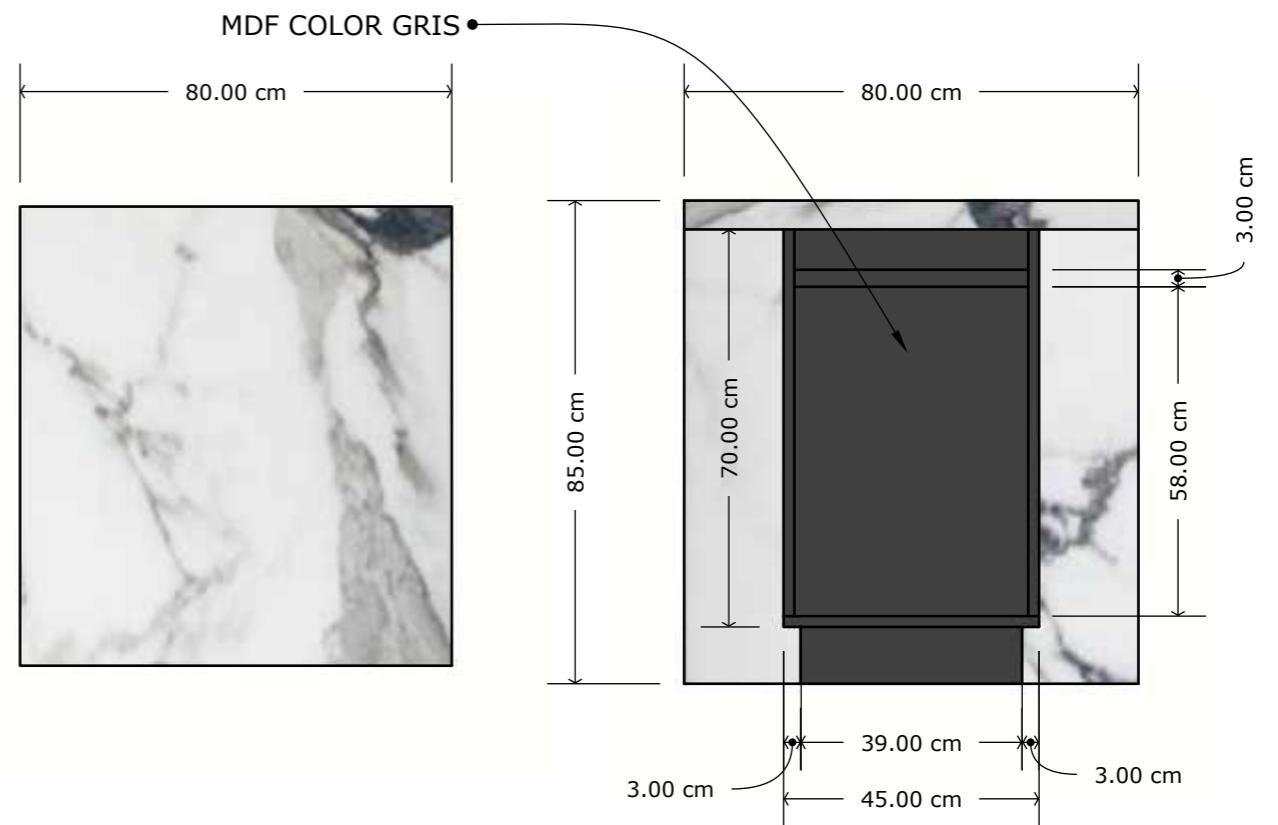
VISTA TRASERA
