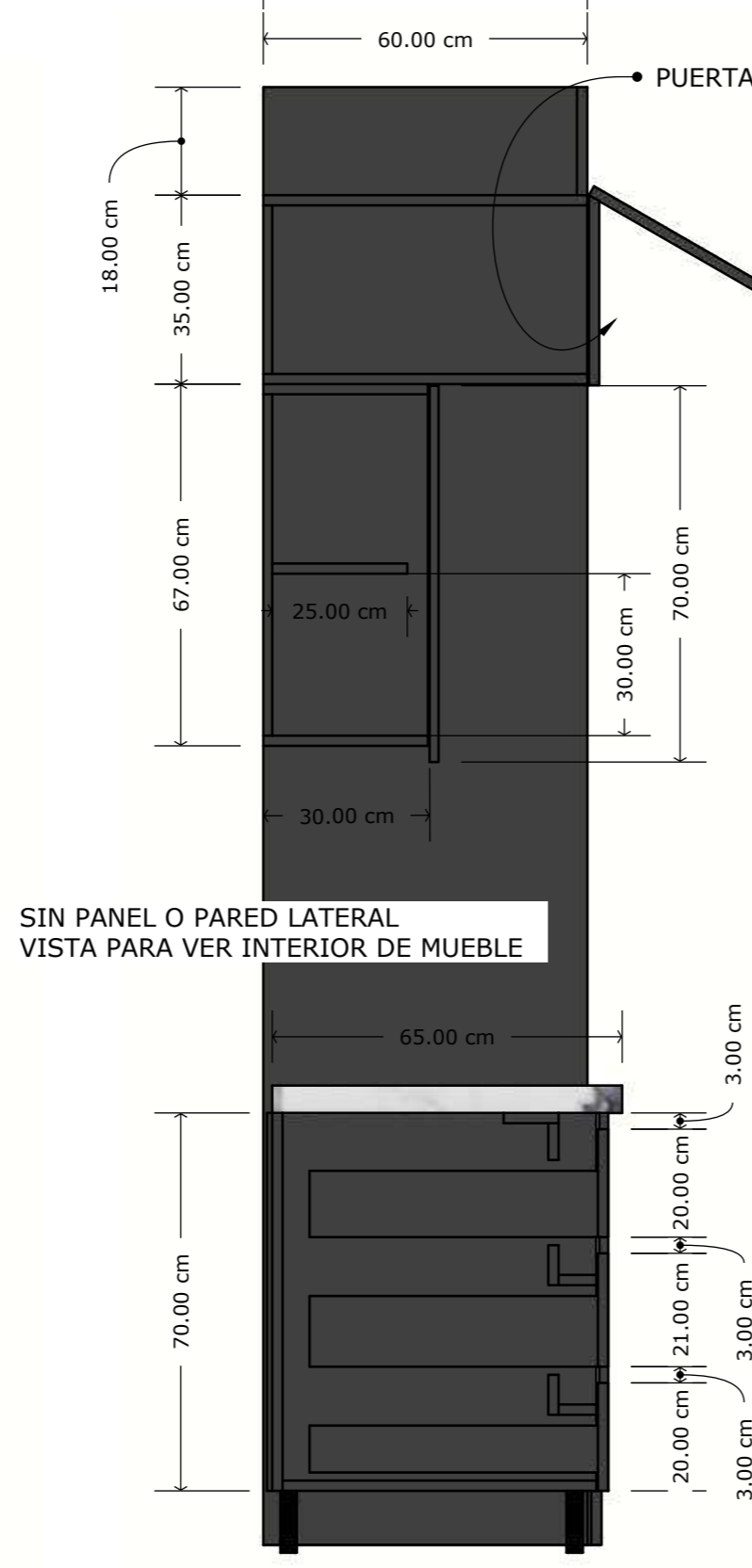
VISTA LATERAL IZQUIERDA MUEBLE 03
