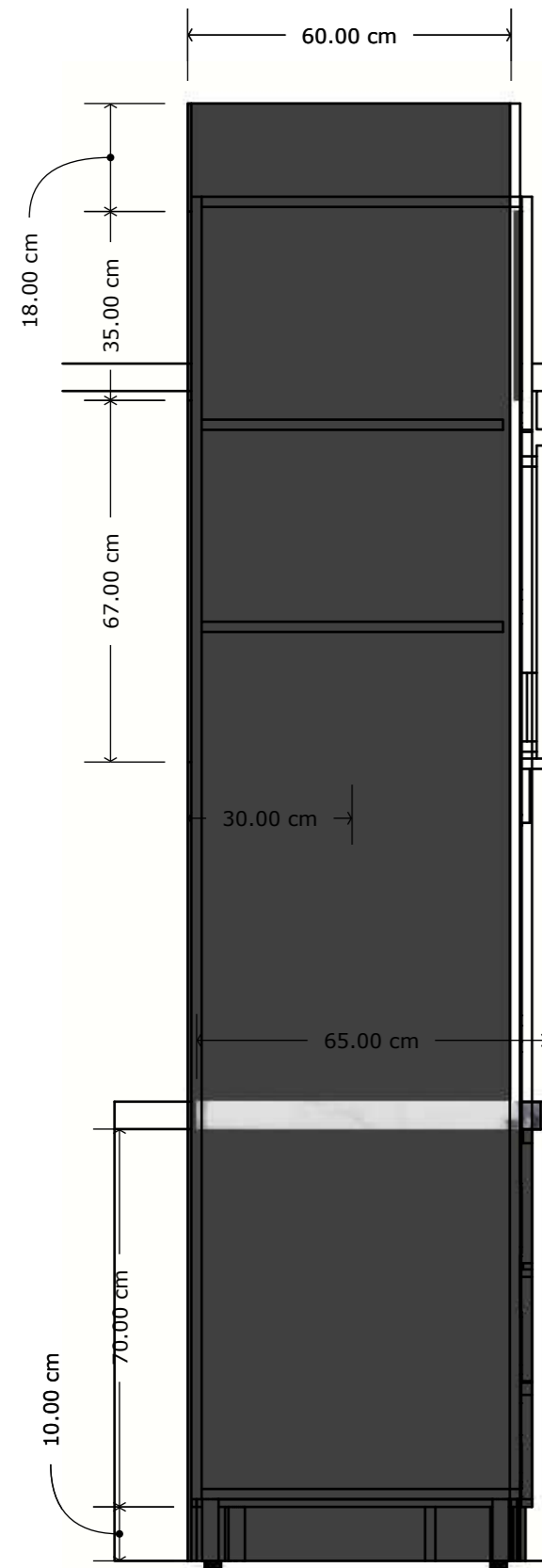
VISTA LATERAL IZQUIERDA MUEBLE 03
