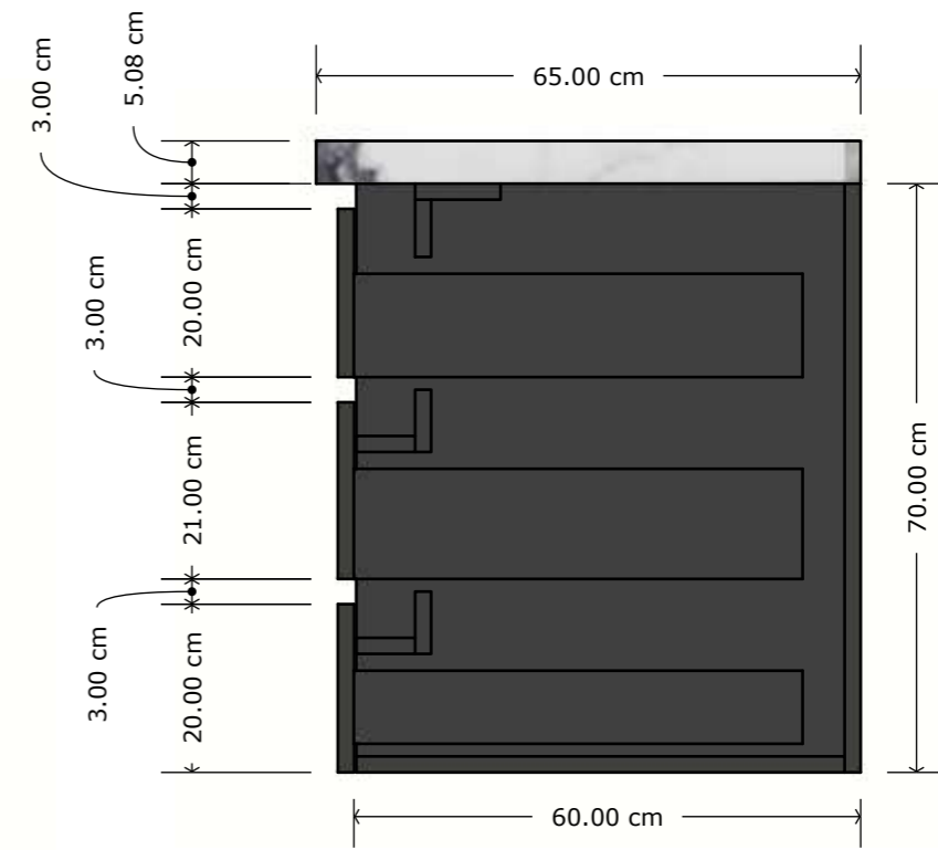
VISTA LATERAL ① ②
