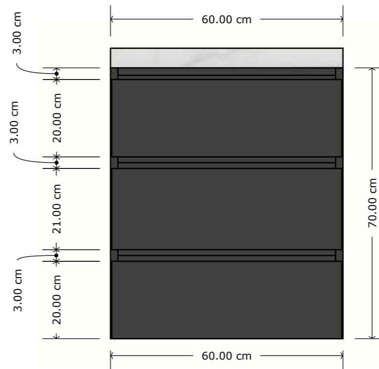
VISTA FRONTAL - FUNCIONAMIENTO Y DIMENSIONES DE GAVETAS
