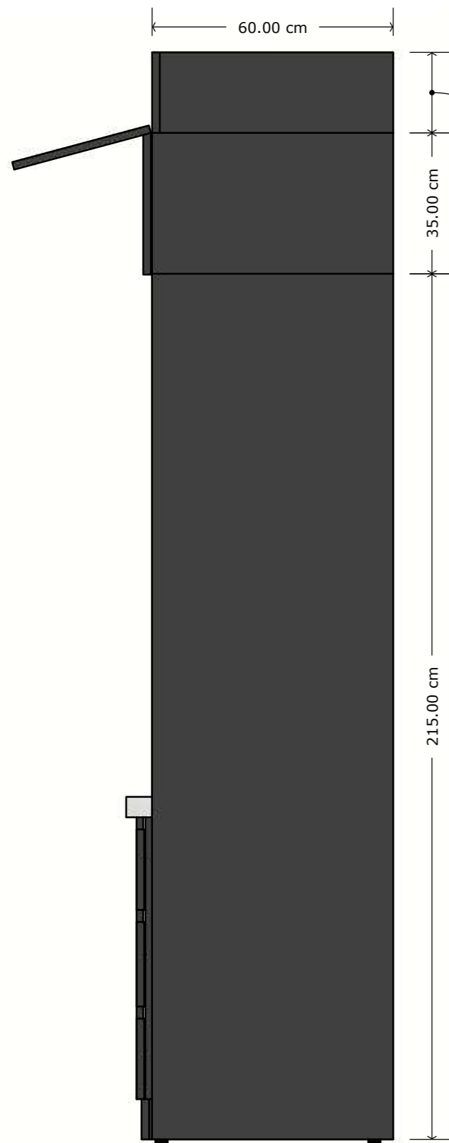
VISTA LATERAL IZQUIERDA MUEBLE 03
