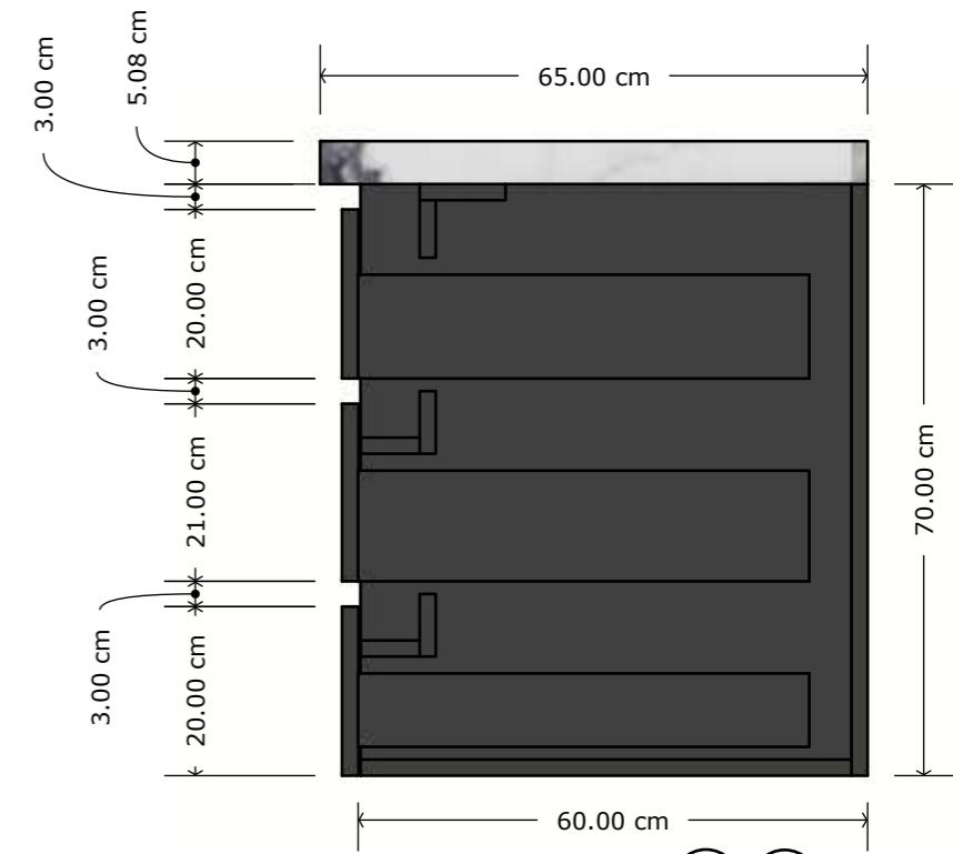
VISTA LATERAL (4) (6)
